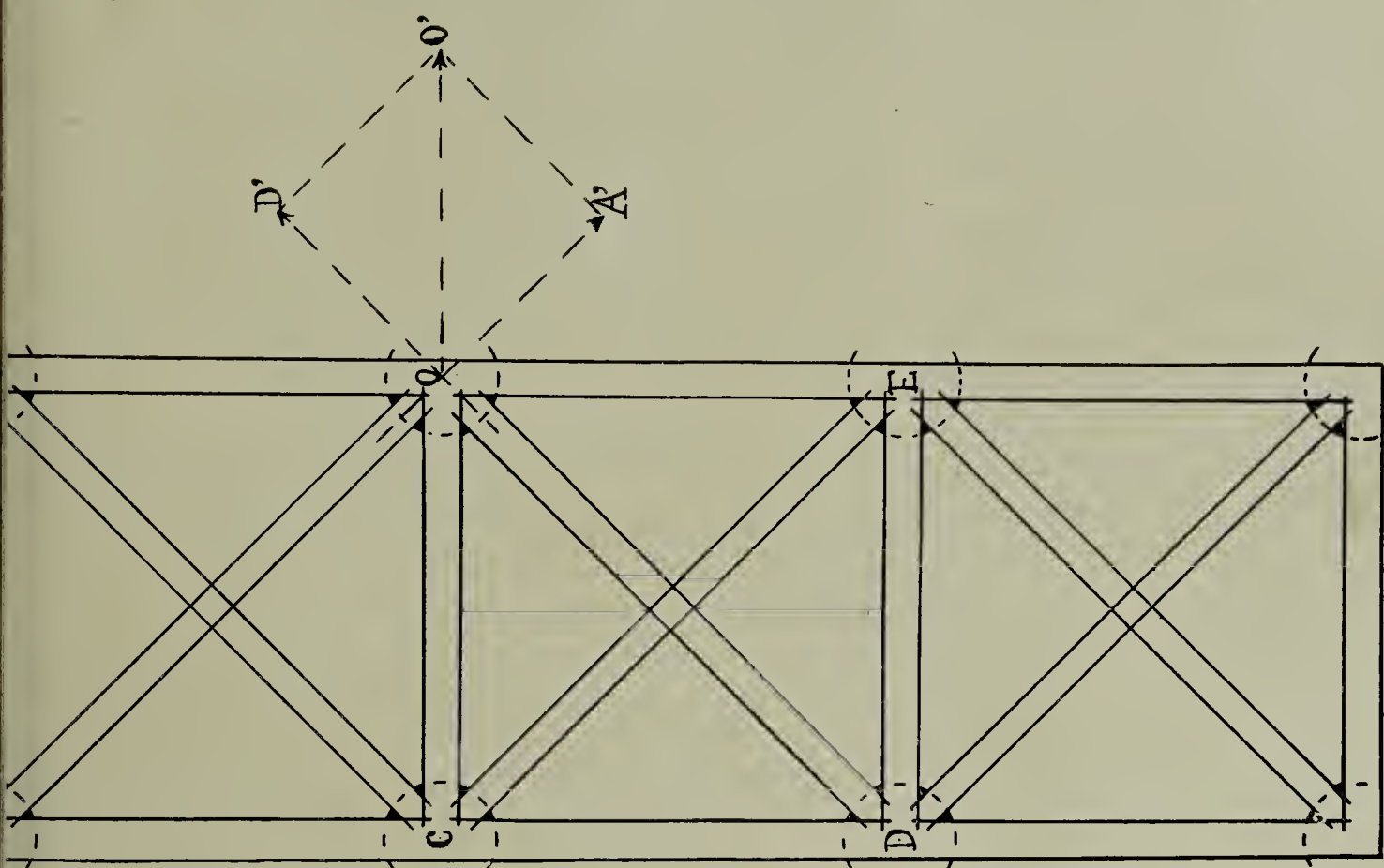
FIGURA 102—Empujes laterales de una bóveda ojival. Proyección horizontal.
